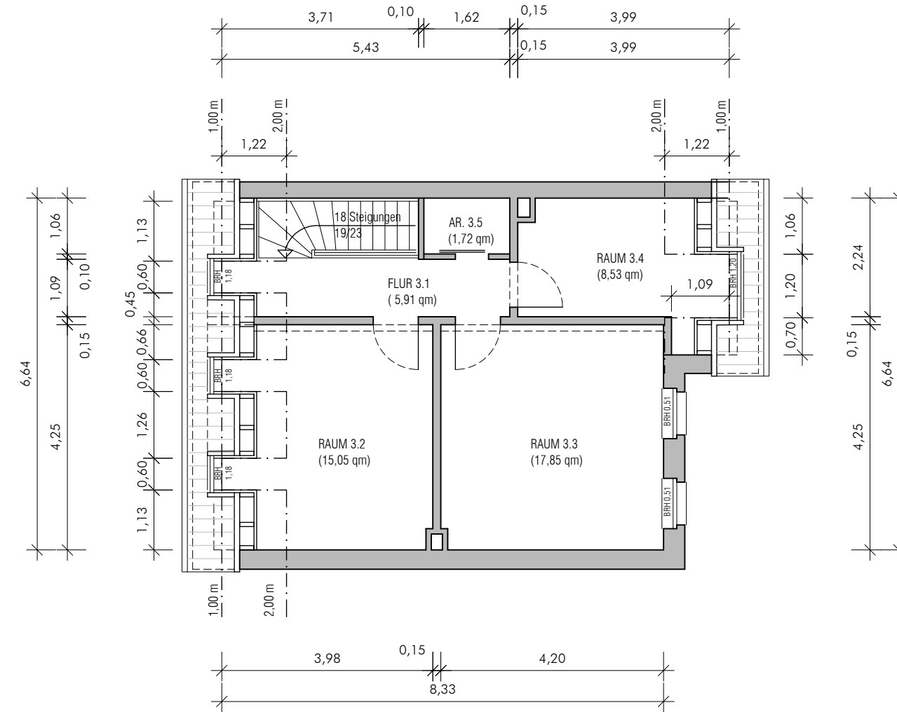
DACHGESCHOSS
